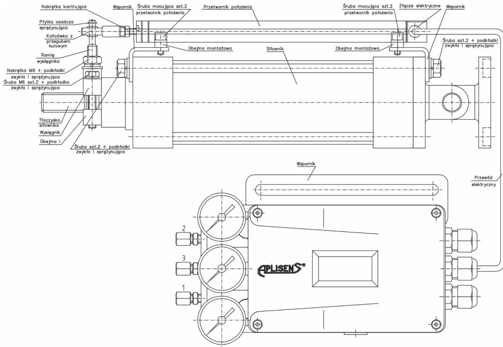
Rys.12. Montaż ustawnika APIS-2X1-..., APIS-2X2-... z zestawem montażowym APIS-XXXX-SS lub SO (ustawnik zabudowany poza siłownikiem dwustronnego działania o ruchu liniowym np.: serii CNOMO produkcji PREMA Kielce lub zgodnym z ISO 6431 (siłowniki produkcji PREMA Kielce lub FESTO).
