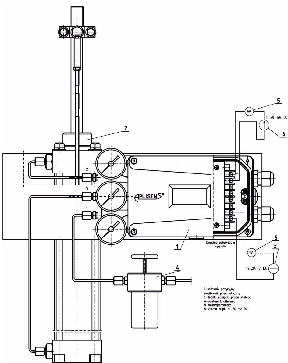
Rys. 20. Schemat układu pomiarowego do uruchomienia ustawnika APIS-2X0... (siłownik liniowy dwustronnego działania)
