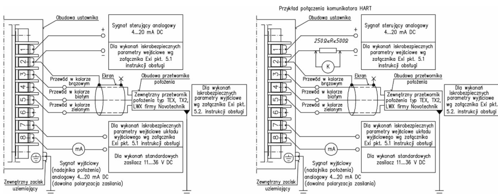
Rys.21d Schemat połączeń elektrycznych ustawnika dla wykonania z zewnętrznym przetwornikiem położenia w warunkach gdy:
