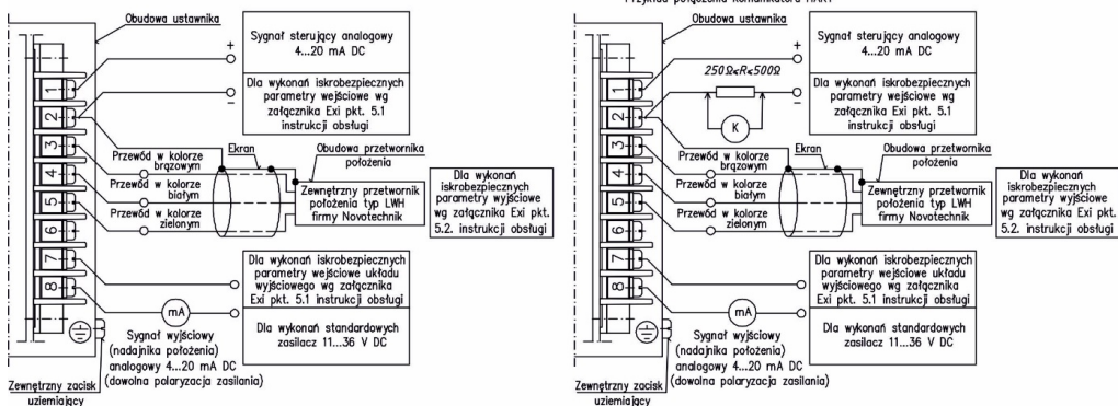
Rys.21c Schemat połączeń elektrycznych ustawnika dla wykonania z zewnętrznym przetwornikiem położenia w warunkach gdy:
