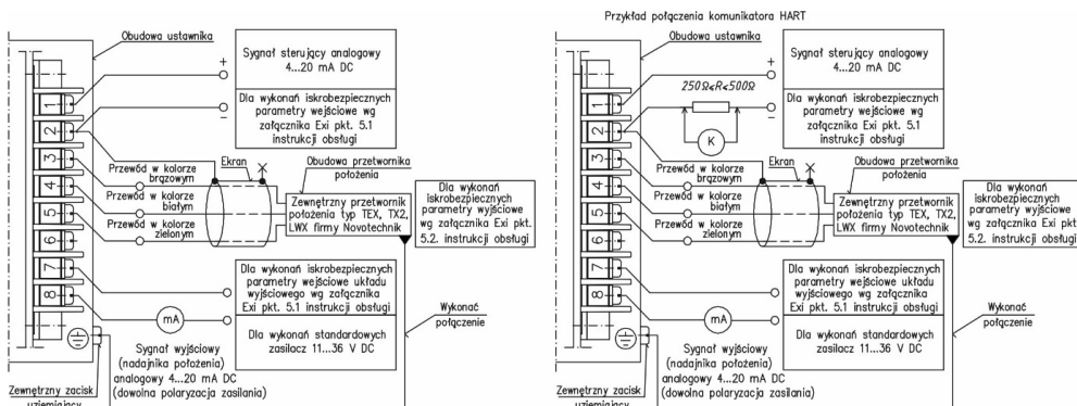
Rys.21b Schemat połączeń elektrycznych ustawnika dla wykonaw z zewnętrznym przetwornikiem położenia w
